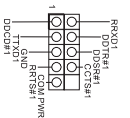
RS-232 Port 4 Pin Headers 15 : COM5 16 : COM6 17 : COM4 18 : COM3
