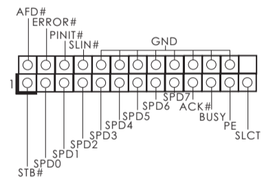
14 : Printer Port Header
